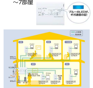
■情報配線システム まとめてねっとギガ+光コンセント付 ~7部屋
