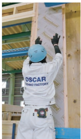
壁断熱材の組込み
